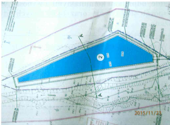
Plan sytuacyjny powyższego zbiornika
